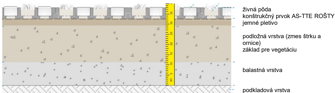
Obrázok č. 3: Zelený systém AS-TTE ROŠTY ® konštrukčný princíp 3
