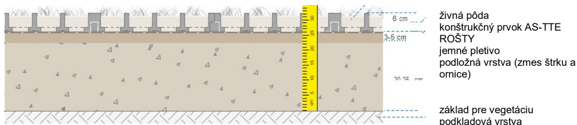
Obrázok č. 2: Zelený systém AS-TTE ROŠTY ® konštrukčný princíp 2
