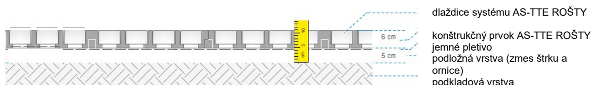
Obrázok č. 4: Spevnený (dláždený) systém AS-TTE ROŠTY ® konštrukčný princíp 1
